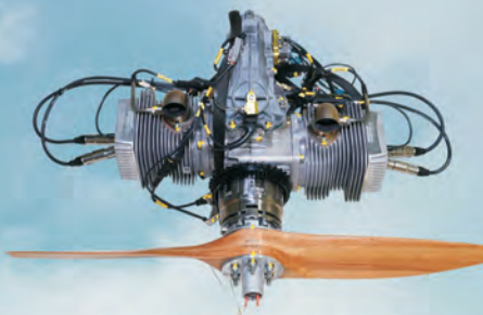
TEI-PG50
